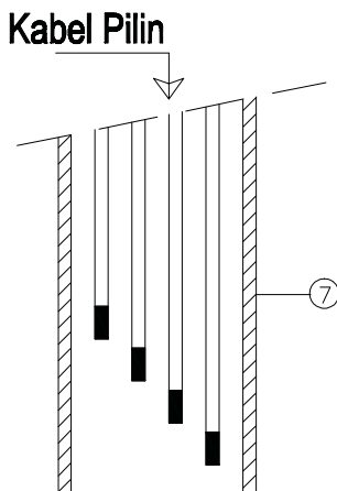
DETAIL dalam pipa DVC
