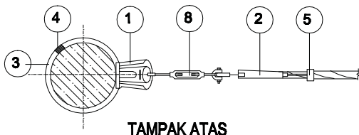
TAMPAK ATAS
