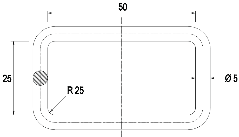
LINK 25 x 50
