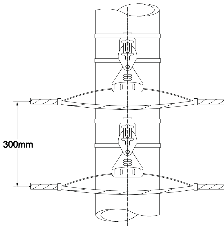
TAMPAK DEPAN
