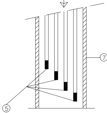
DETAIL dalam pipa DVC
