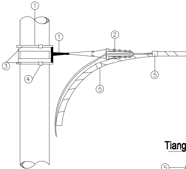
konstruksi FDE pada tiang awal
