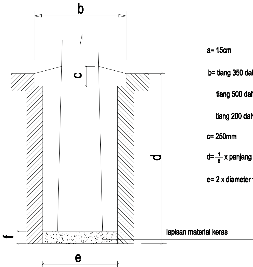
PONDASI TIPE-D
