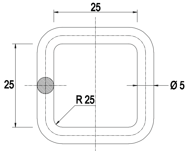
LINK 25 x 25
