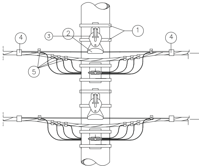
TAMPAK DEPAN
