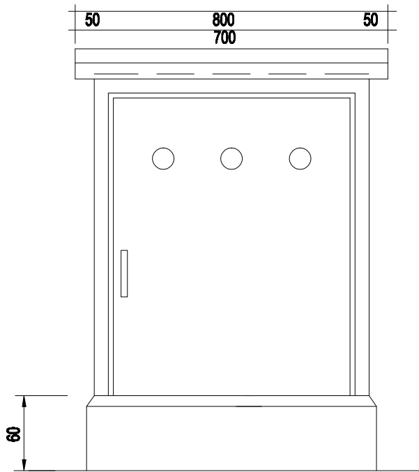
TAMPAK MUKA
