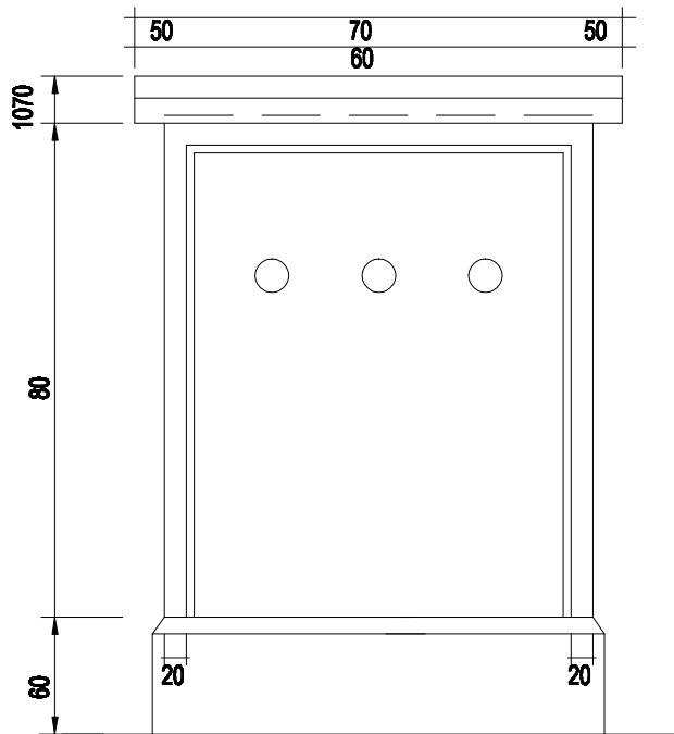
TAMPAK MUKA
