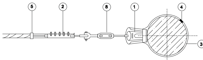
TAMPAK ATAS
